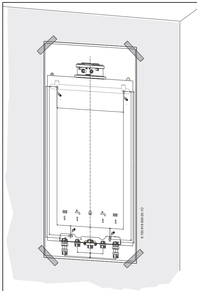
Rys. 9 Szablon montażowy
