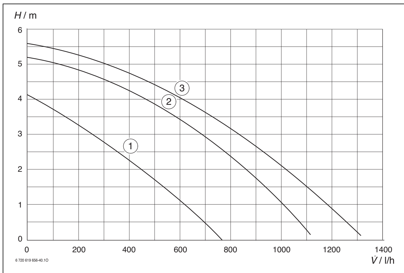
Rys. 34 Charakterystyka pompy
