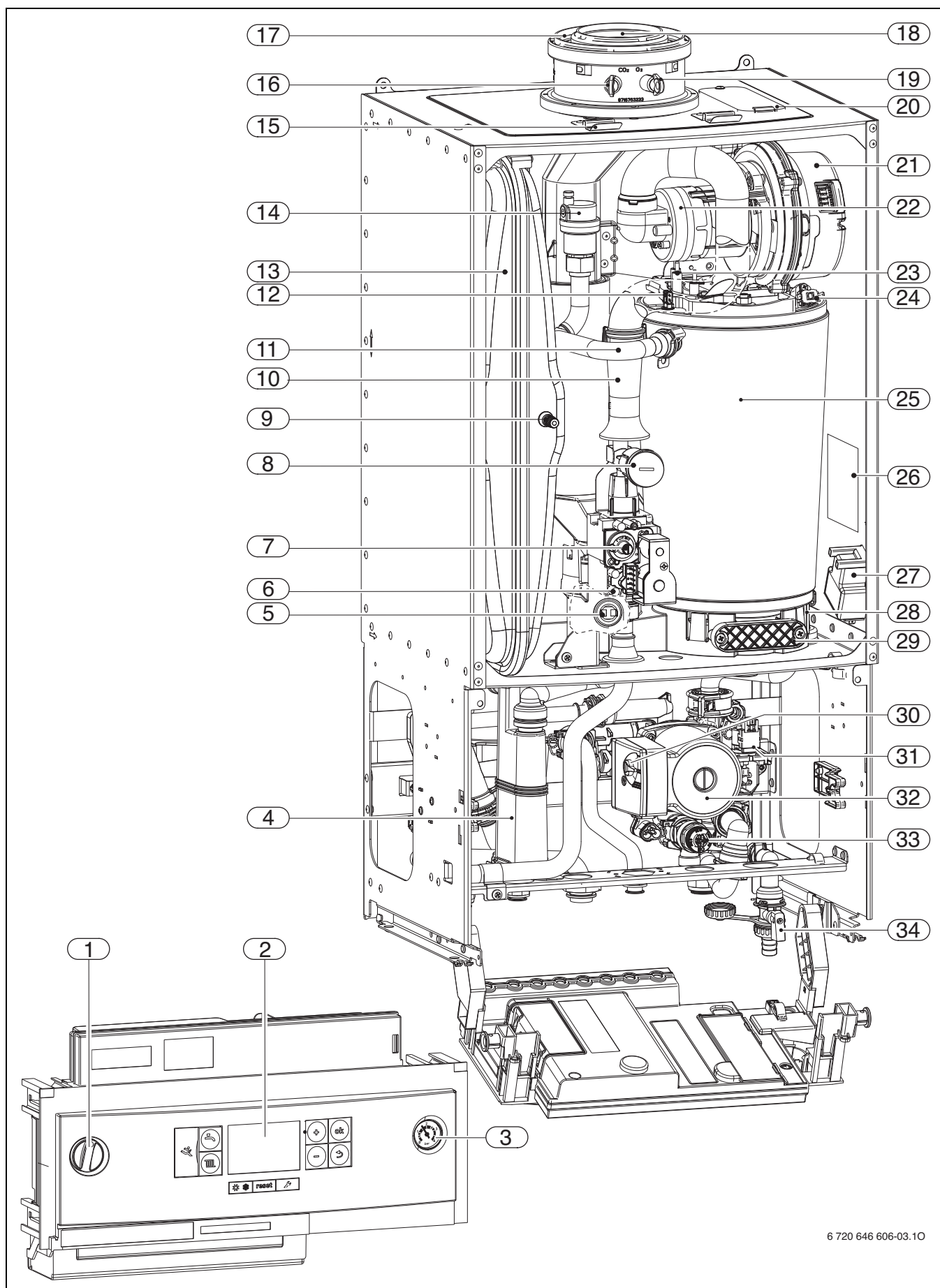
Rys. 5 GB072-14/20/24
