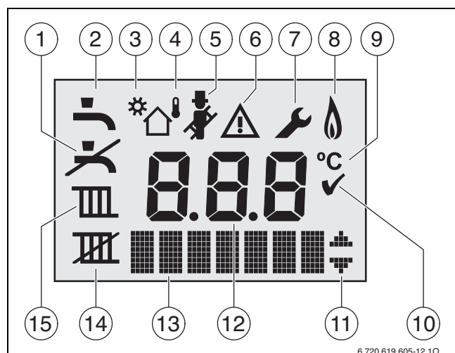
Rys. 6 Wskazania wyświetlacza
