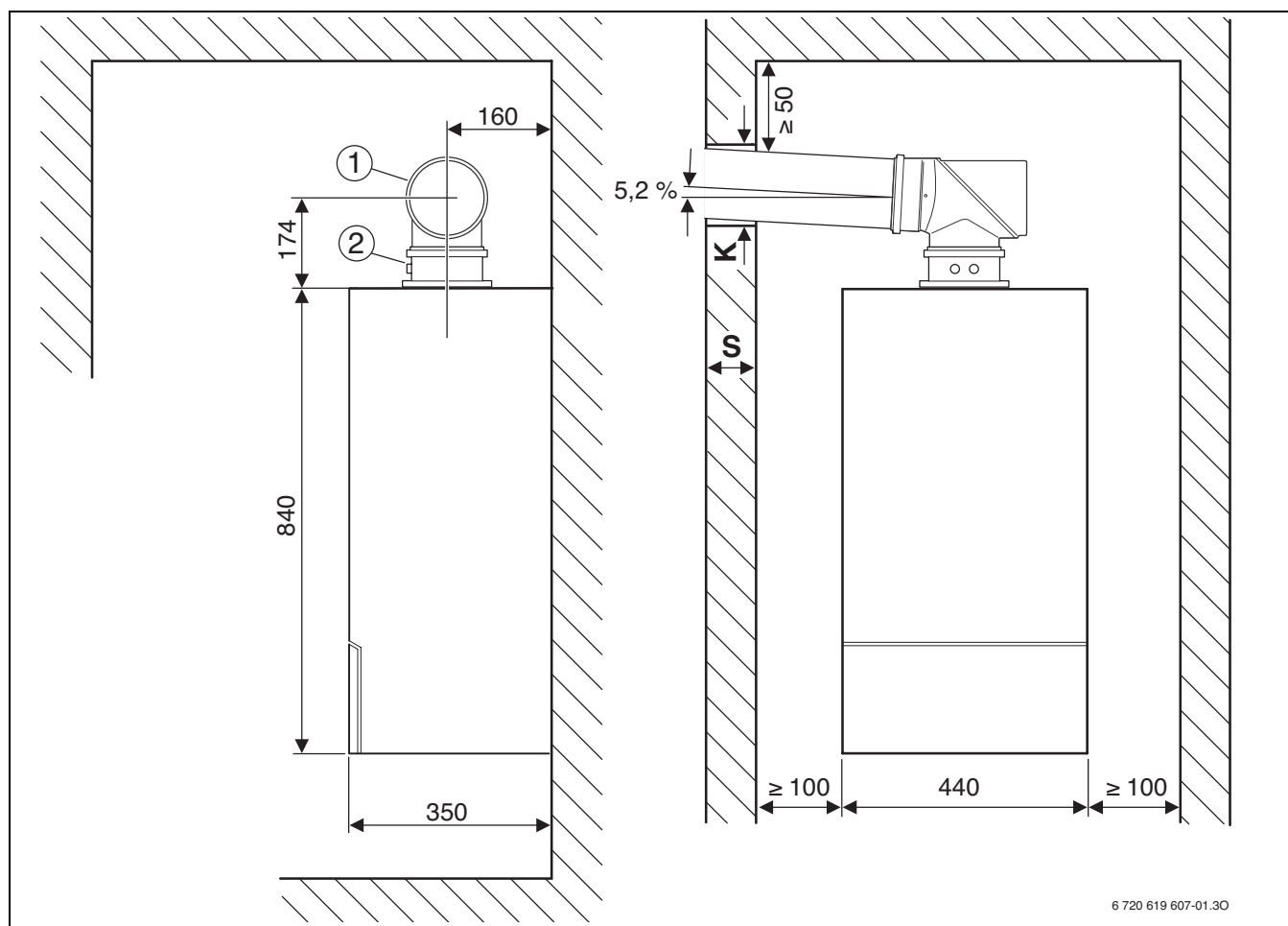
Rys. 8 Odprowadzenie spalin Ø 80/125 mm lub Ø 80 mm
