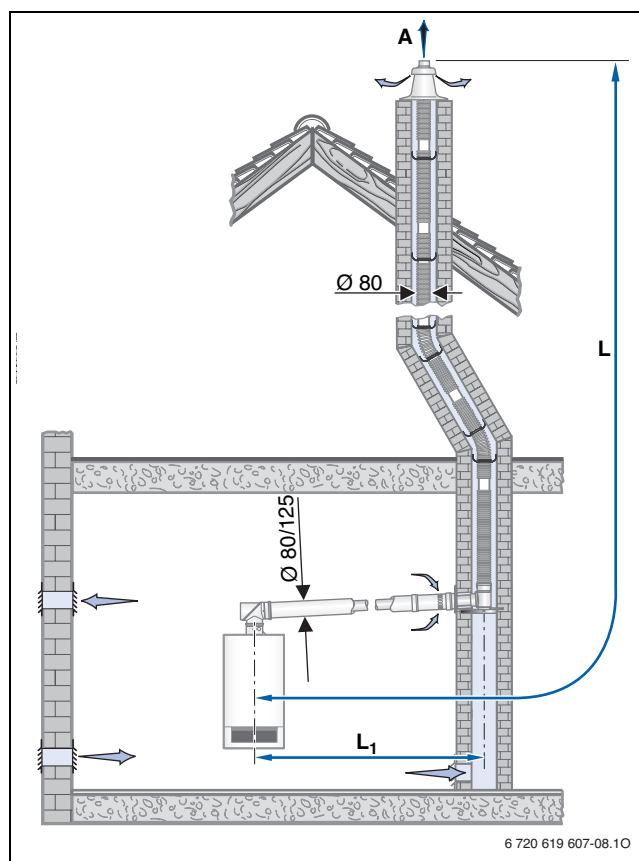
Rys. 15 Wariant montażu przy użyciu zestawu montażowego GA-X + GA-K + ÜB-Flex
