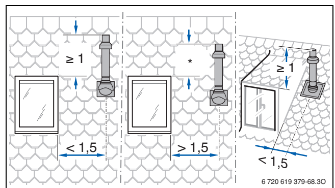
Rys. 3 Minimalne odległości od okien w przypadku zestawu DO (przykłady wg MuFeuVO); (wymiary w m)
