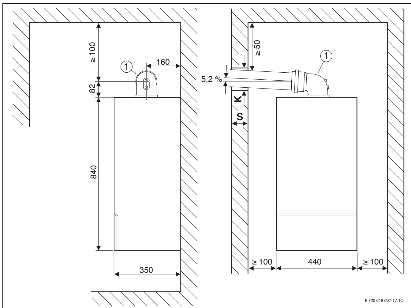
Rys. 9 Odprowadzenie spalin Ø 60/100 mm
