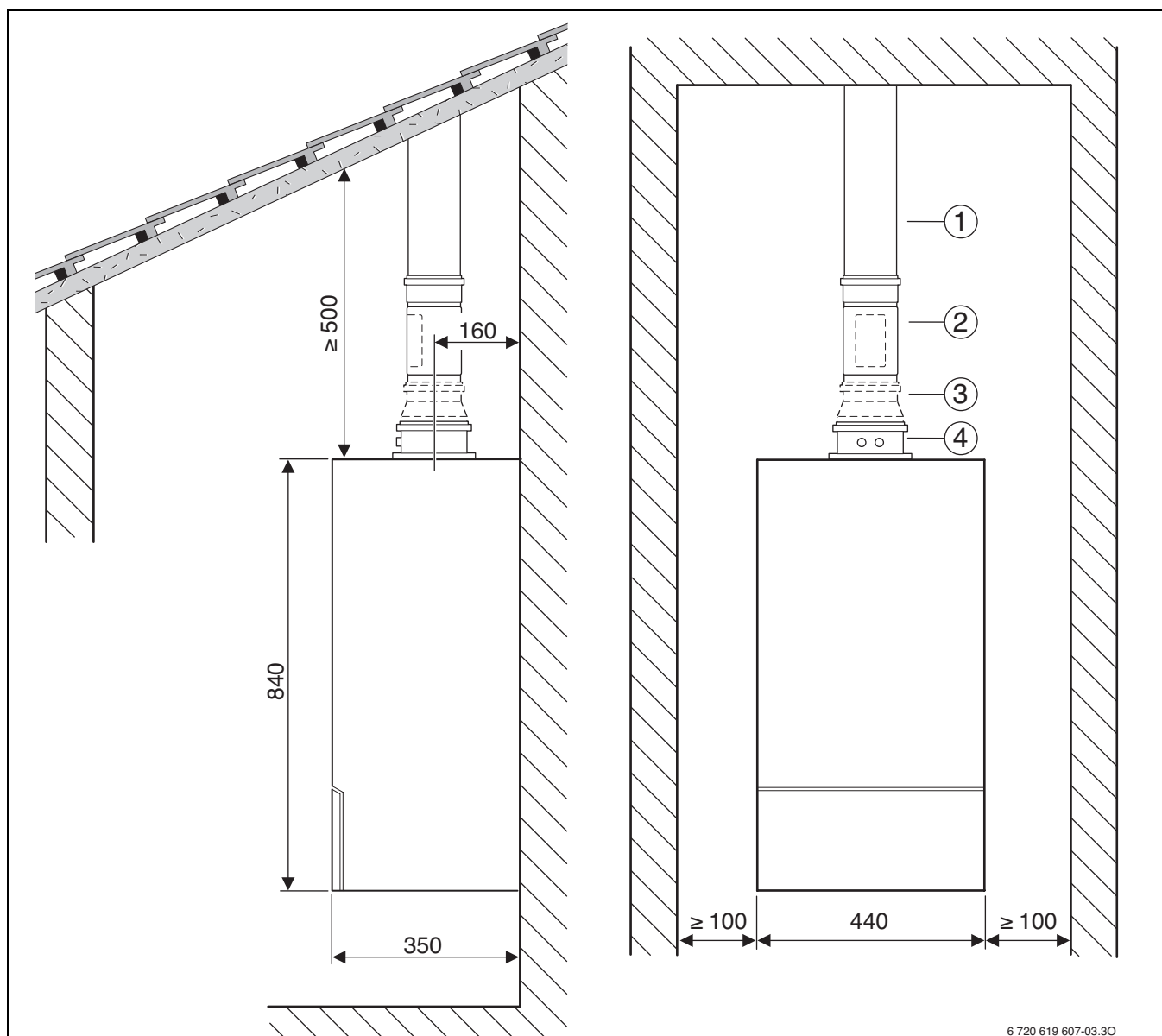
Rys. 11 Dach skośny
