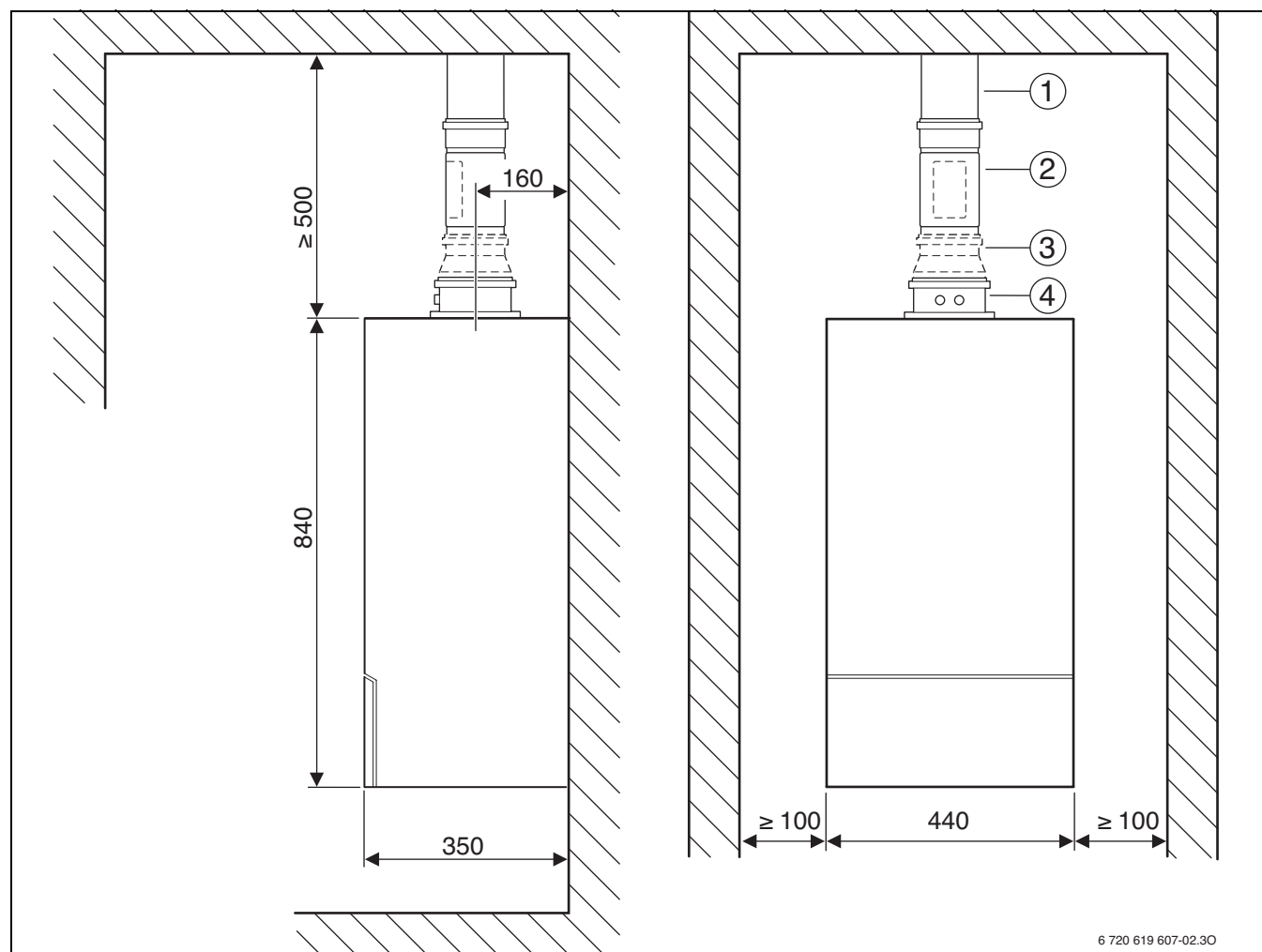
Rys. 10 Dach płaski
