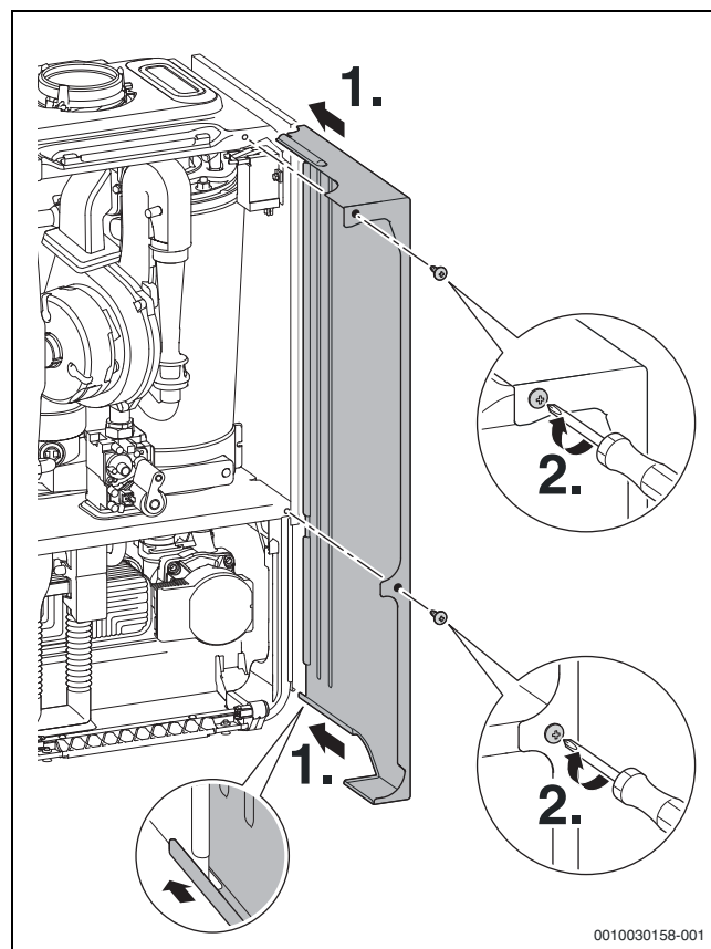
Rys. 79 Ponowne zakładanie obudowy bocznej
