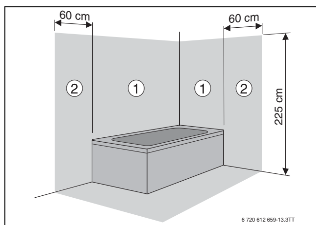
Rys. 37 Strefy ochronne
