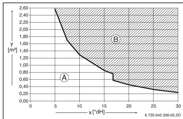
Rys. 30 Wymagania dotyczące wody do napełniania i uzupełniania w °dH do urządzeń o mocy < 50 kW
