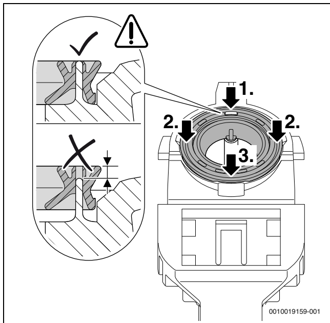
Rys. 65 Docisnięcie uszczelki
