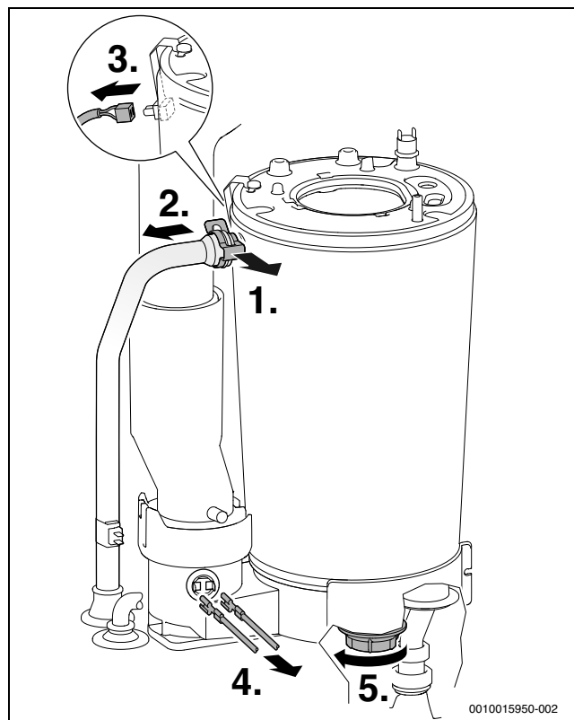
Rys. 75 Odtwarzanie rury zasilania i kabla
