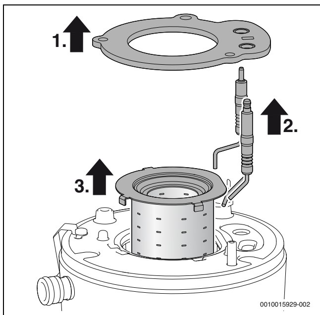
Rys. 55 Wyjmowanie palnika
