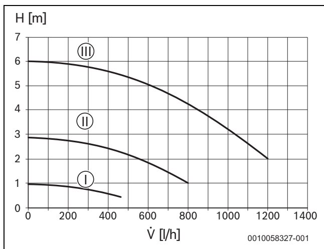
Rys. 45 Charakterystyka pompy c.o. (stałe ciśnienie)
