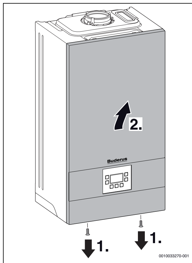
Rys. 33 Zdjęcie przedniej obudowy
