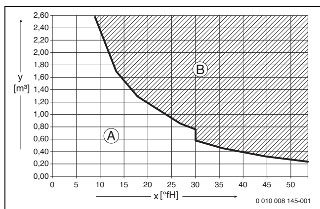
Rys. 31 Wymagania dotyczące wody do napełniania i uzupełniania w ^{\circ}\text{FH} do urządzeń o mocy < 50 \text{ kW}
