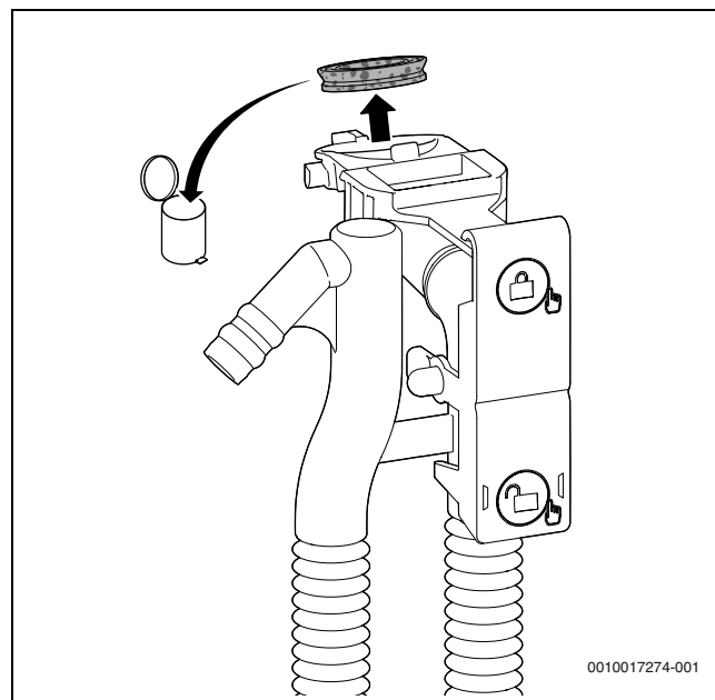
Rys. 63 Wymiana uszczelki u góry na syfonie kondensatu
