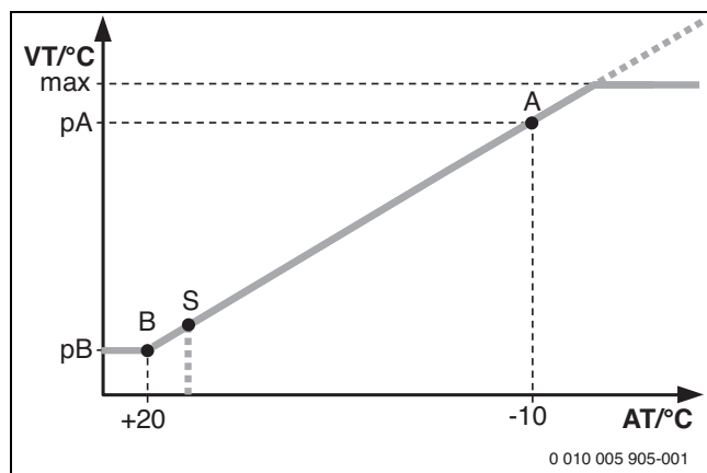
Rys. 83 Krzywa grzewcza
