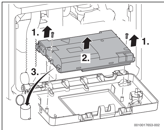
Rys. 77 Zdejmowanie pokrywy i wymiana płyty głównej
