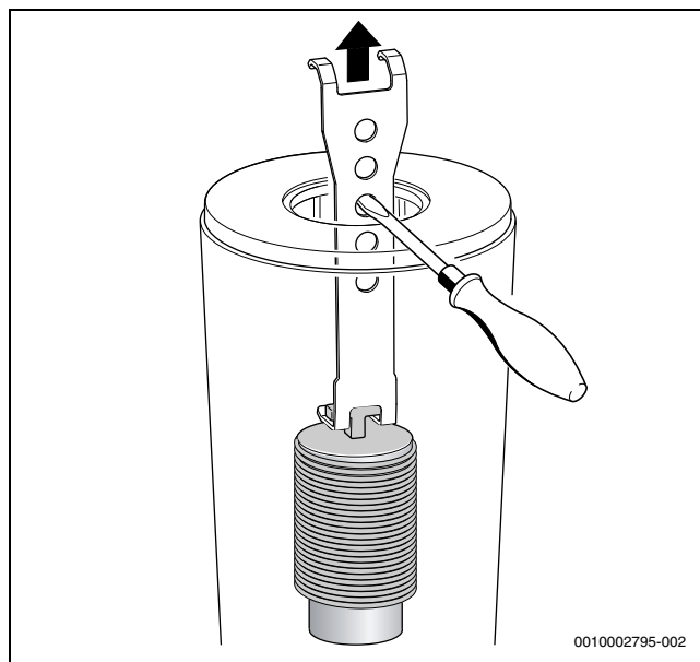
Rys. 57 Wyjmowanie dolnego elementu waporowego
