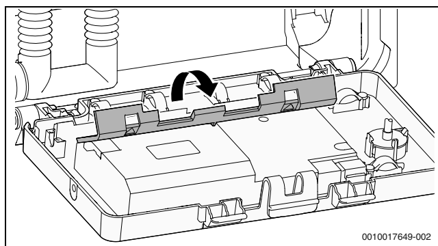
Rys. 39 Otwieranie pokrywy
