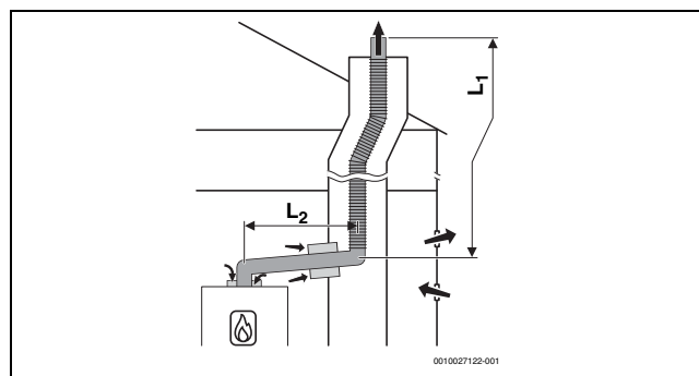
Rys. 17 Elastyczne odprowadzenie spalin w szachcie wg B_{23p}/B_{53p} z zależnym od powietrza w pomieszczeniu doprowadzeniem powietrza do urządzenia i koncentryczną złączką między pomieszczeniem zainstalowania a szachtem
