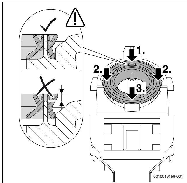
Rys. 59 Docisnięcie uszczelki
