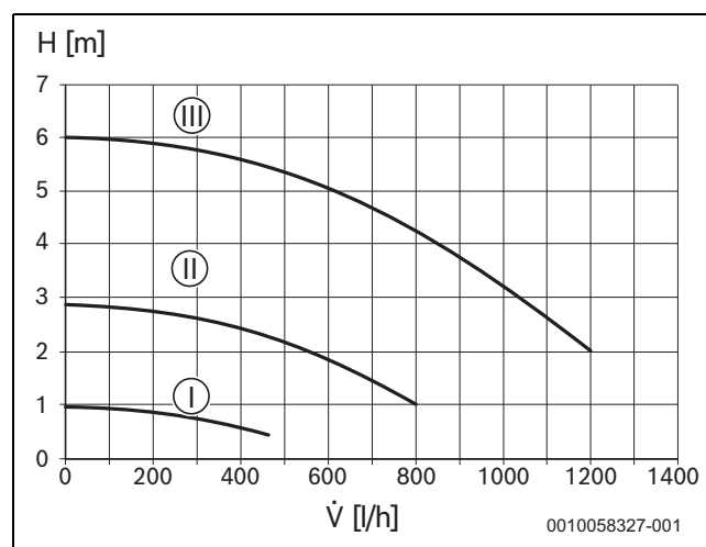
Rys. 38 Charakterystyka pompy c.o. (stałe ciśnienie)
