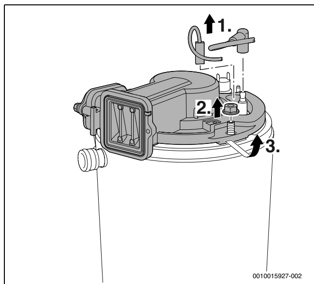
Rys. 47 Odłączenie pokrywy palnika
