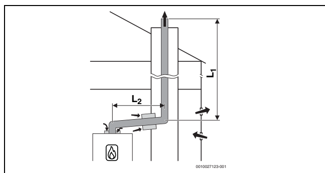
Rys. 16 Sztywne odprowadzenie spalin w szachcie wg B_{23p}/B_{53p} z zależnym od powietrza w pomieszczeniu doprowadzeniem powietrza do urządzenia i koncentryczną złączką między pomieszczeniem zainstalowania a szachtem
