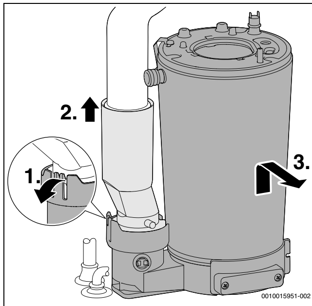
Rys. 70 Demontaż bloku ciepłego
