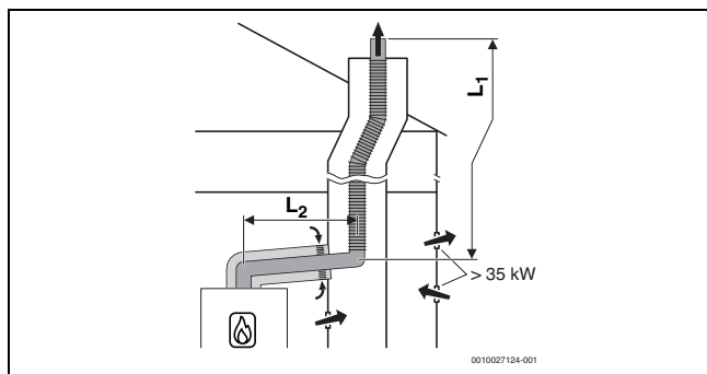
Rys. 19 Elastyczne odprowadzenie spalin wg B 33 z zależnym od powietrza w pomieszczeniu doprowadzeniem powietrza przez koncentryczną instalację powietrzno-spalinową w pomieszczeniu zainstalowania
