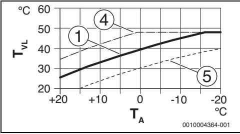
Rys. 11 Ustawienie krzywej grzewczej dla ogrzewania podłogowego Przesunięcie równoległe powyżej zadanej temperatury w pomieszczeniu
