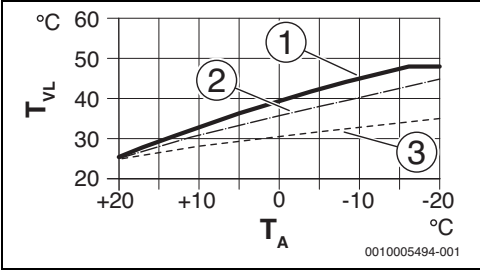
Rys. 10 Ustawienie krzywej grzewczej dla ogrzewania podłogowego Wzrost powyżej temperatury projektowej T_{AL} i minimalnej temperatury zewnętrznej T_{A,min} .
