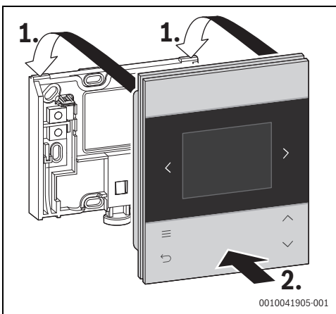
Rys. 7 Zawieszenie sterownika
