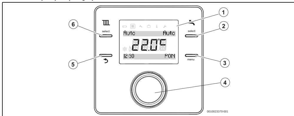
Rys. 1 Sterownik
