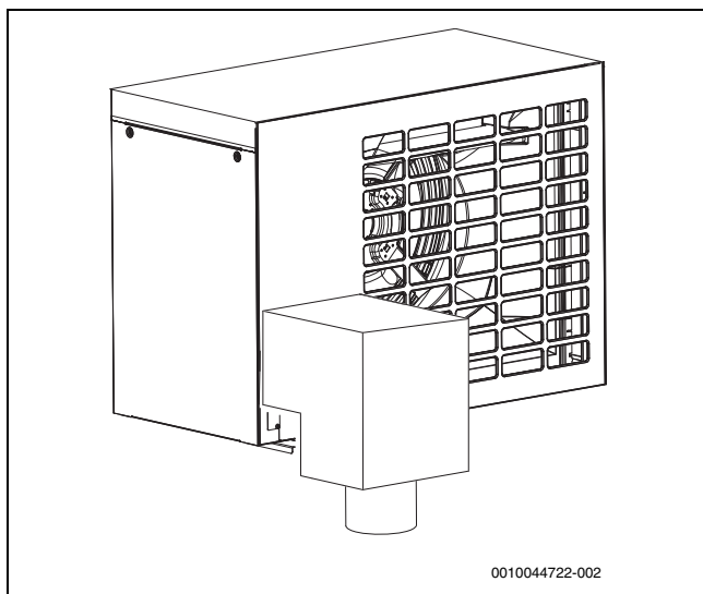
Rys. 27 Zestaw montażowy, montaż na podłodze
