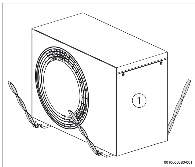
Rys. 16 Używanie pasów do transportu pompy ciepła bez opakowania
