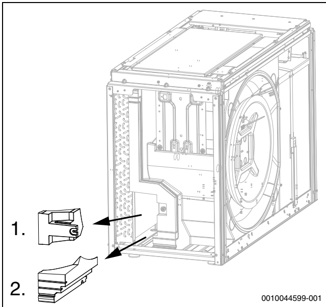
Rys. 48 Części EPP
