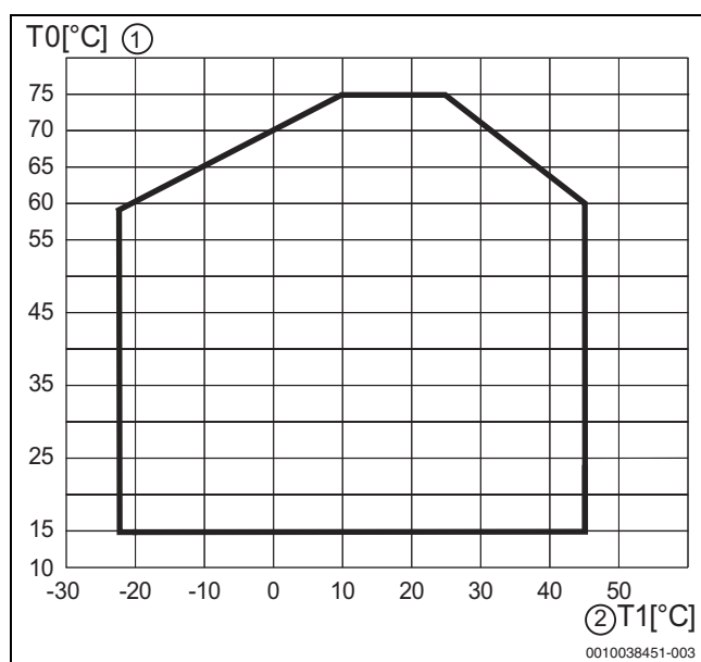
Rys. 51 Pompa ciepła w trybie grzania, bez dogrzewacza
