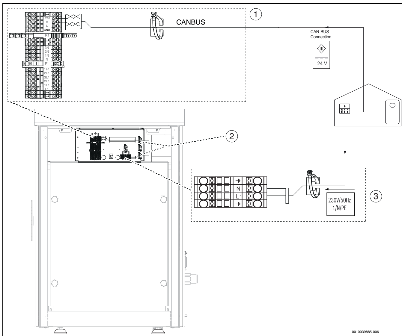
Rys. 44 Skrzynka zaciskowa
