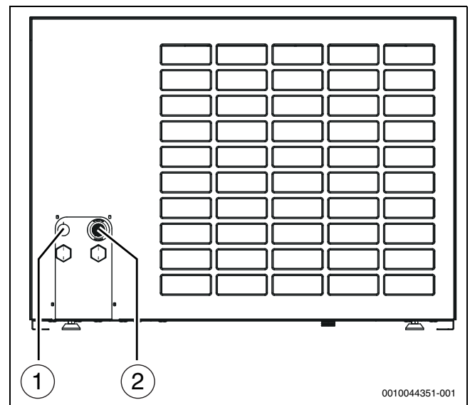
Rys. 43 Kanały kablowe
