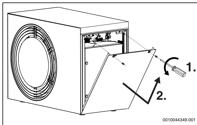
Rys. 38 Ośłona boczna
