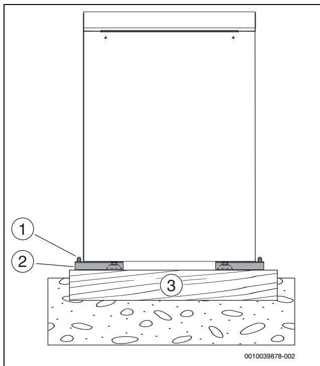
Rys. 25 Przytworzenie pompy ciepła
