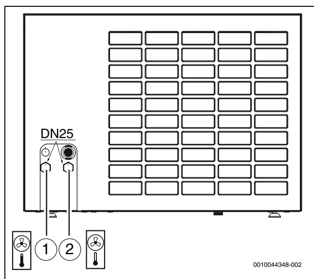
Rys. 37 Łączniki rurowe nośnika ciepła; opis dotyczy wszystkich rozmiarów
