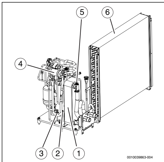
Rys. 3 Przegląd produktu, widok z tyłu
