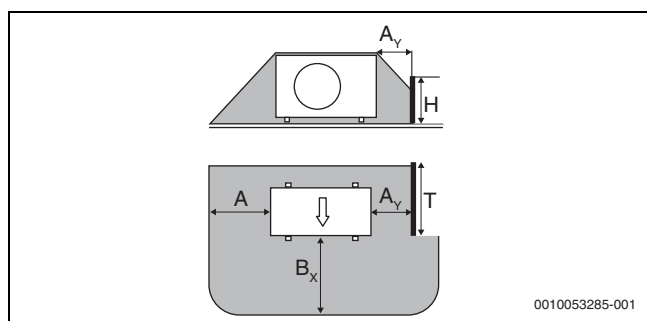
Rys. 9 Obszar bezpieczeństwa z barierą po prawej stronie, podłogowo-stojąca pompa ciepła
