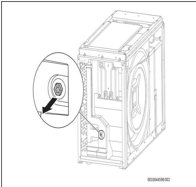
Rys. 47 Odkręcanie
