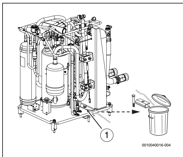
Rys. 40 Śruba transportowa
