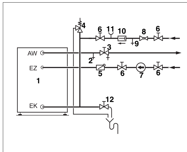
Rys. 7 Instalacja wg DIN 1988 (widok ogólny)
