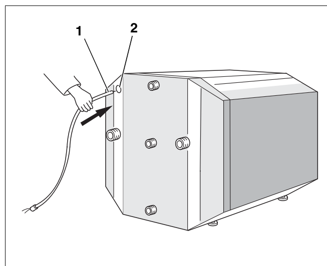
Rys. 9 Montaż czujnika temperatury
