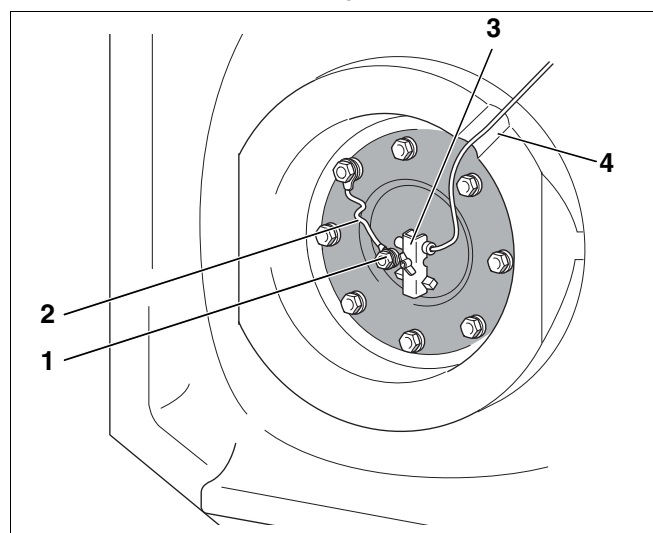
Rys. 10 Sprawdzenie przyłącza anody magnezowej
